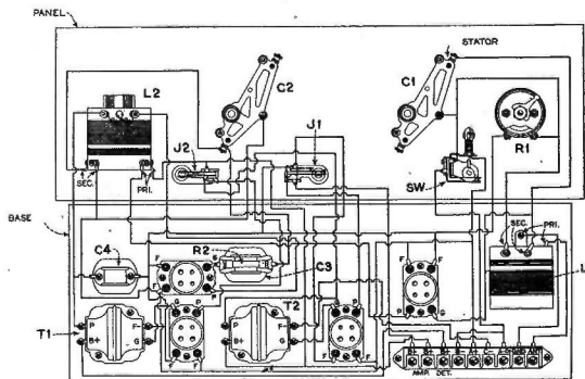
Un paso de radio, detector "tres circuitos" y dos pasos de audio.
