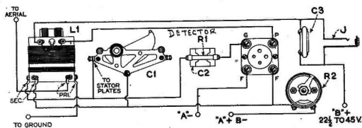
Circuito detector solo
